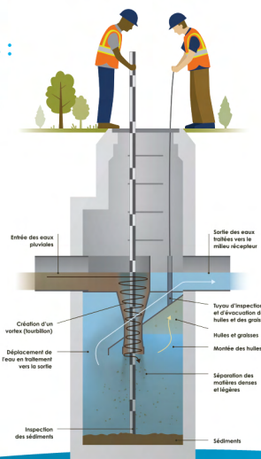
COUPE TRANSVERSALE D'UN CAPTEUR DE SÉDIMENTS
